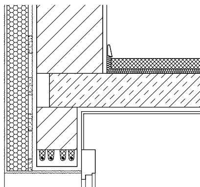
Оконная перемычка с наружной тепловой изоляцией
