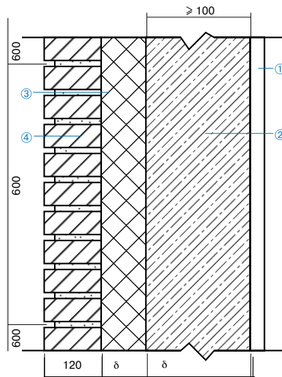
Рис. 2. Трехслойная стена.
