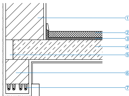
Существующая теплоизолированная оконная перемычка
