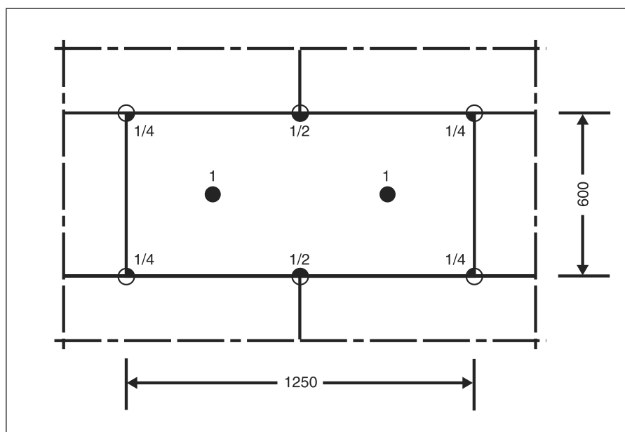
Рис. 1. Крепление плит.
