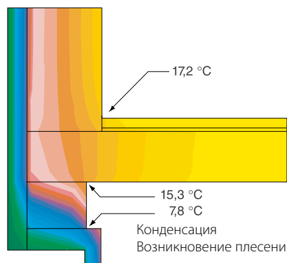
Расположение изотерм у оконной перемычки с наружной теплоизоляцией, опасность конденсации и возникновения плесени
