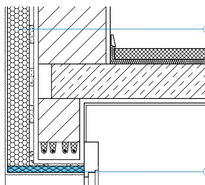
Оконная перемычка с наружной тепловой изоляцией
