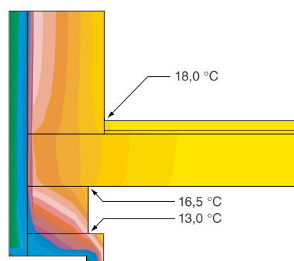
Расположение изотерм при теплоизолированном проеме: без конденсации, нет опасности возникновения плесени
